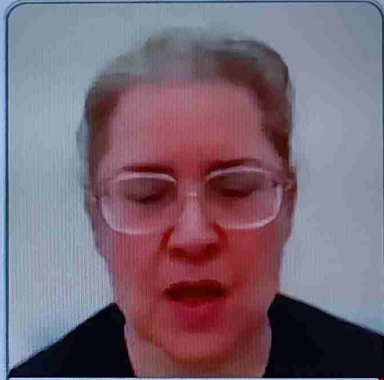
صدیقه وسمقی
